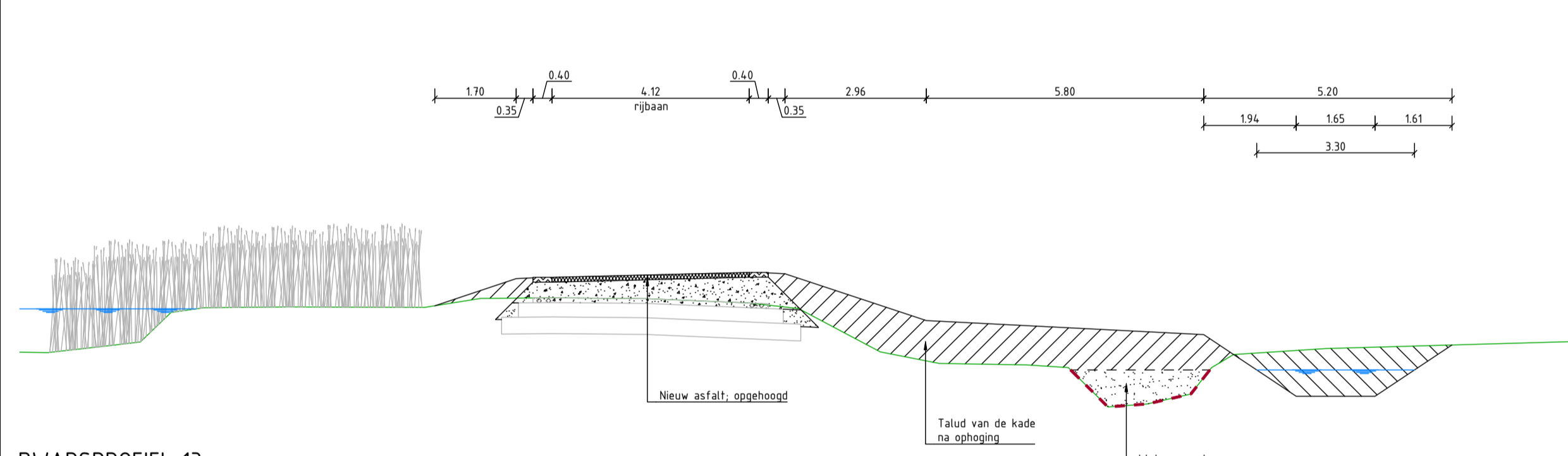
DWARSPROFIEL 13 schaal 1:100
