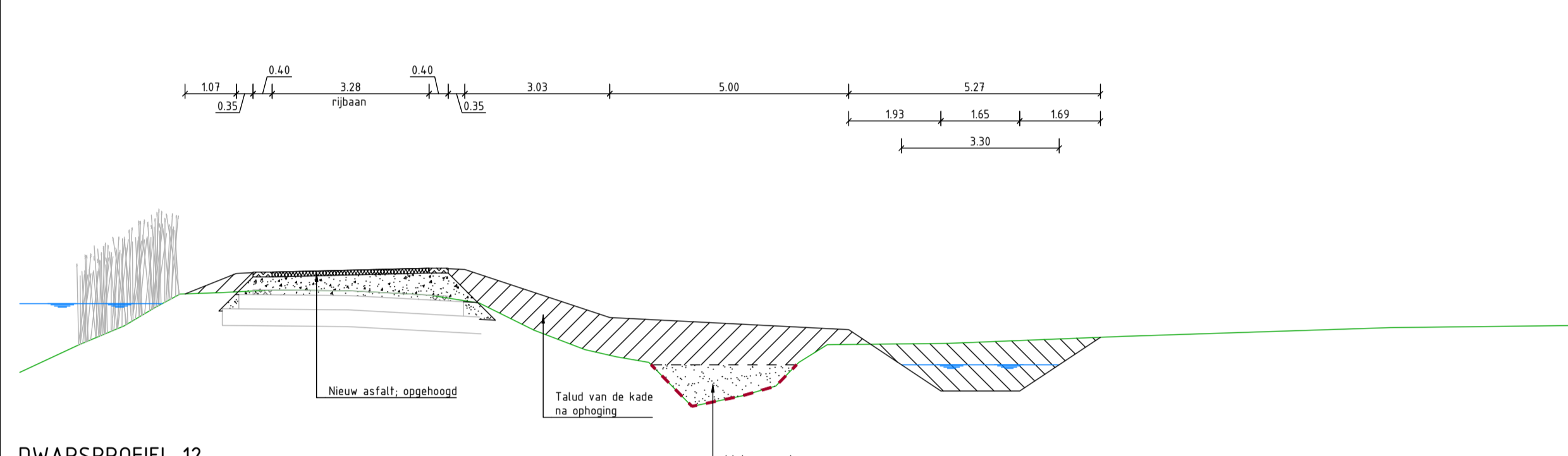
DWARSPROFIEL 12 schaal 1:100
